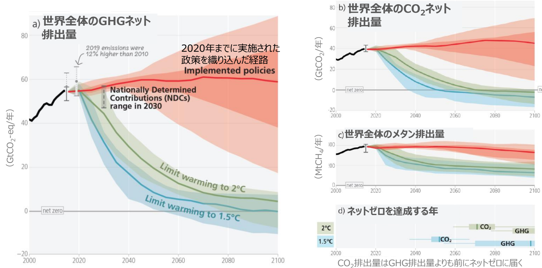
将来の温暖化水準に応じた世界の排出経路
